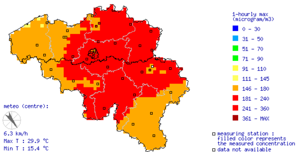
Figuur 6: Hoogste ozonconcentraties op 25 juli 2012.
