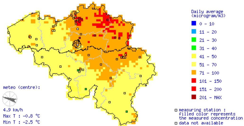
Figuur 5: Daggemiddelde fijnstofconcentratie op 30 januari 2012.
