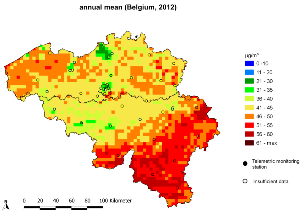
Figuur 47: Ruimtelijke spreiding van de \text{O}_3 -jaargemiddelde concentraties in België, 2012. ‘Insufficient data’ betekent dat de data niet voldoen aan de criteria uit richtlijn 2008/50/EG annex VII voor het aggregeren van de meetgegevens. Alle data werden berekend op basis van de RIO-interpolatietechniek.
