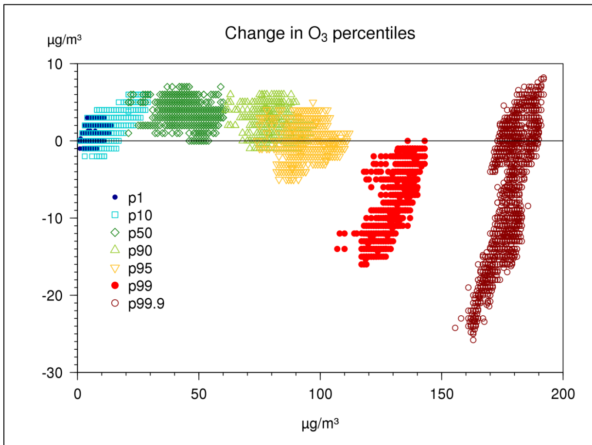
Figuur 52. Verandering in O 3 -percentielen tussen de periode 1990-2001 en 2002-2012 in functie van de percentielwaarden in de periode 2002-2012 voor alle RIO-gridcellen. De data (uurgemiddelde ozonconcentraties) werden gegenereerd op basis van de RIO-interpolatietechniek. De verschillende kleuren geven de verschillende percentielwaarden aan
