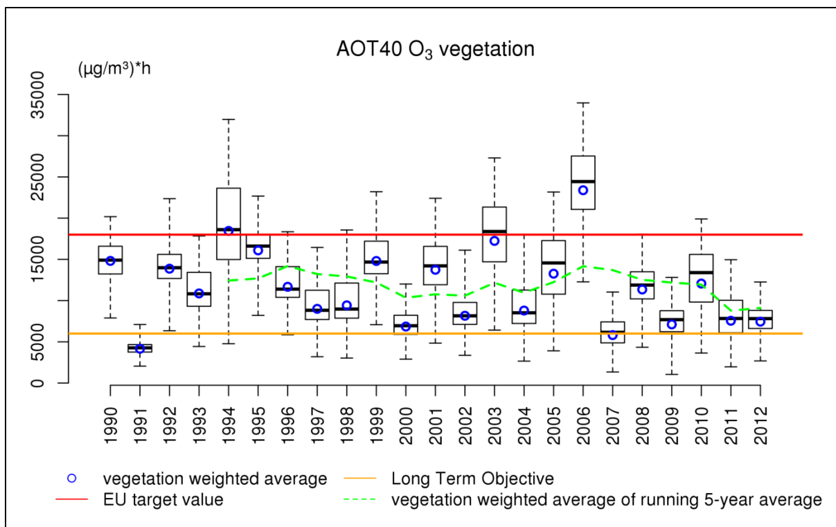
Figuur 44: Boxplots van de overlast voor de vegetatie (AOT40) in België (1990-2012). De vegetatiegewogen gemiddelden voor België worden weergegeven door de blauwe cirkels. De groene stippellijn geeft het vegetatiegewogen gemiddelde weer van de 5-jaargemiddelde AOT40. Alle data werden berekend op basis van de RIO-interpolatietechniek.
