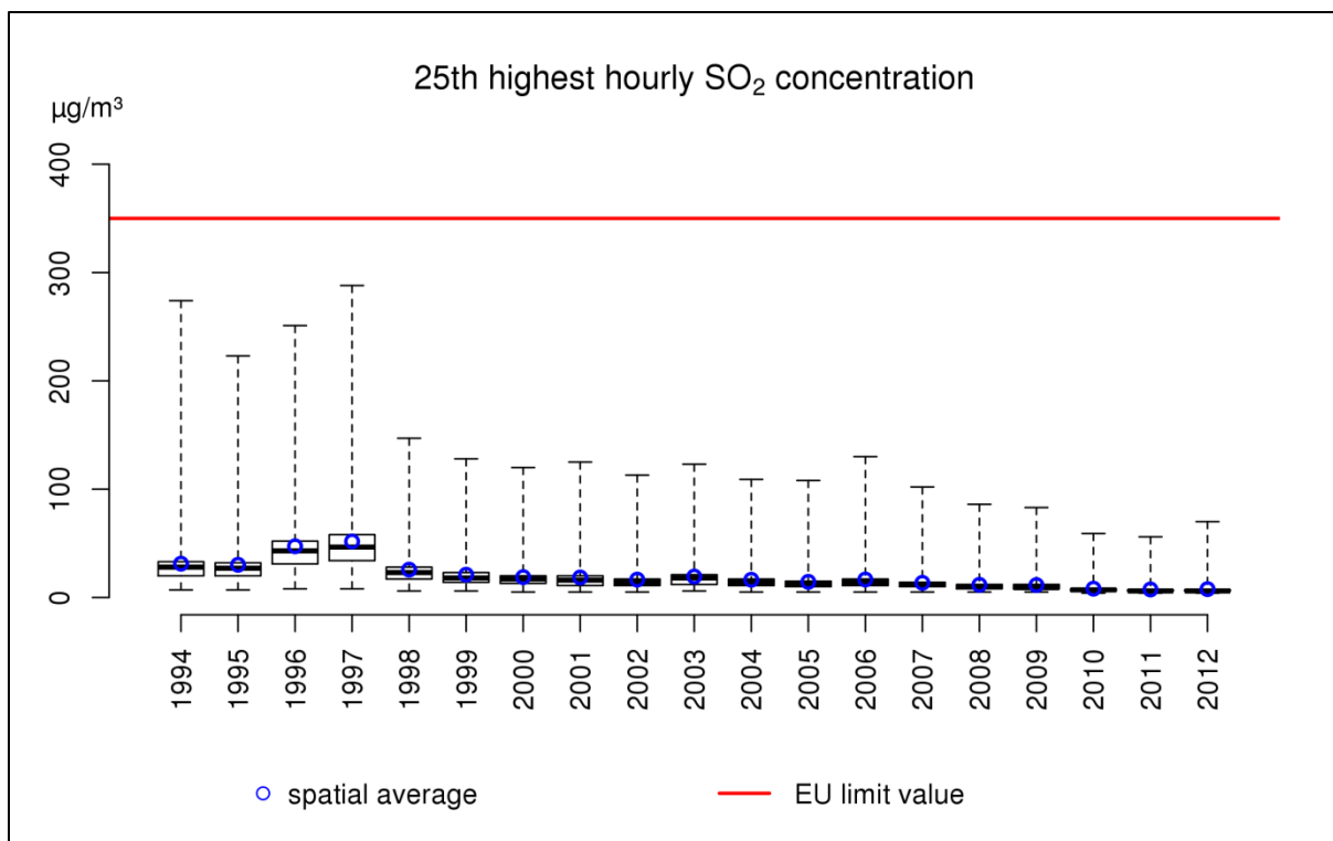
Figuur 55: Boxplot van de 25e hoogste uurgemiddelde SO 2 -concentratie over de periode 1994-2012 in België op basis van de RIO-interpolatietechniek.
