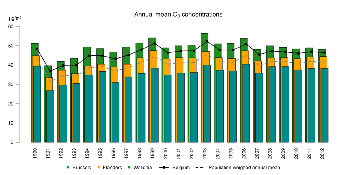
Figuur 50: Evolutie van de jaargemiddelde concentratie in België en de drie gewesten op basis van de RIO-interpolatietechniek.
