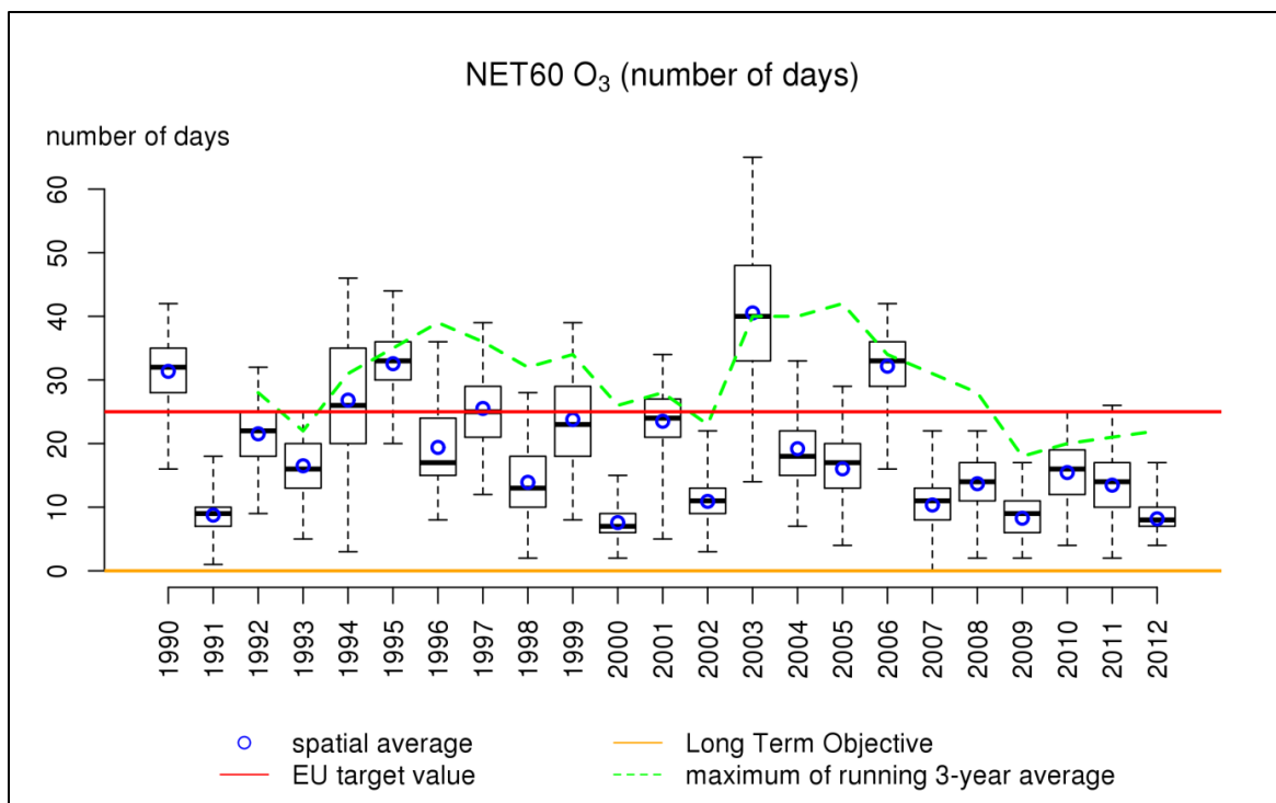
Figuur 38: Boxplots van aantal dagen met hoogste 8-uurgemiddelde ozonconcentraties > 120 µg/m 3 in België in de periode 1990-2012. Het ruimtelijke gemiddelde wordt weergegeven door de blauwe cirkels. De groene stippellijn geeft het maximum van het 3-jaargemiddelde aantal overschrijdingsdagen in België weer. Alle data werden berekend op basis van de RIO-interpolatietechniek.
