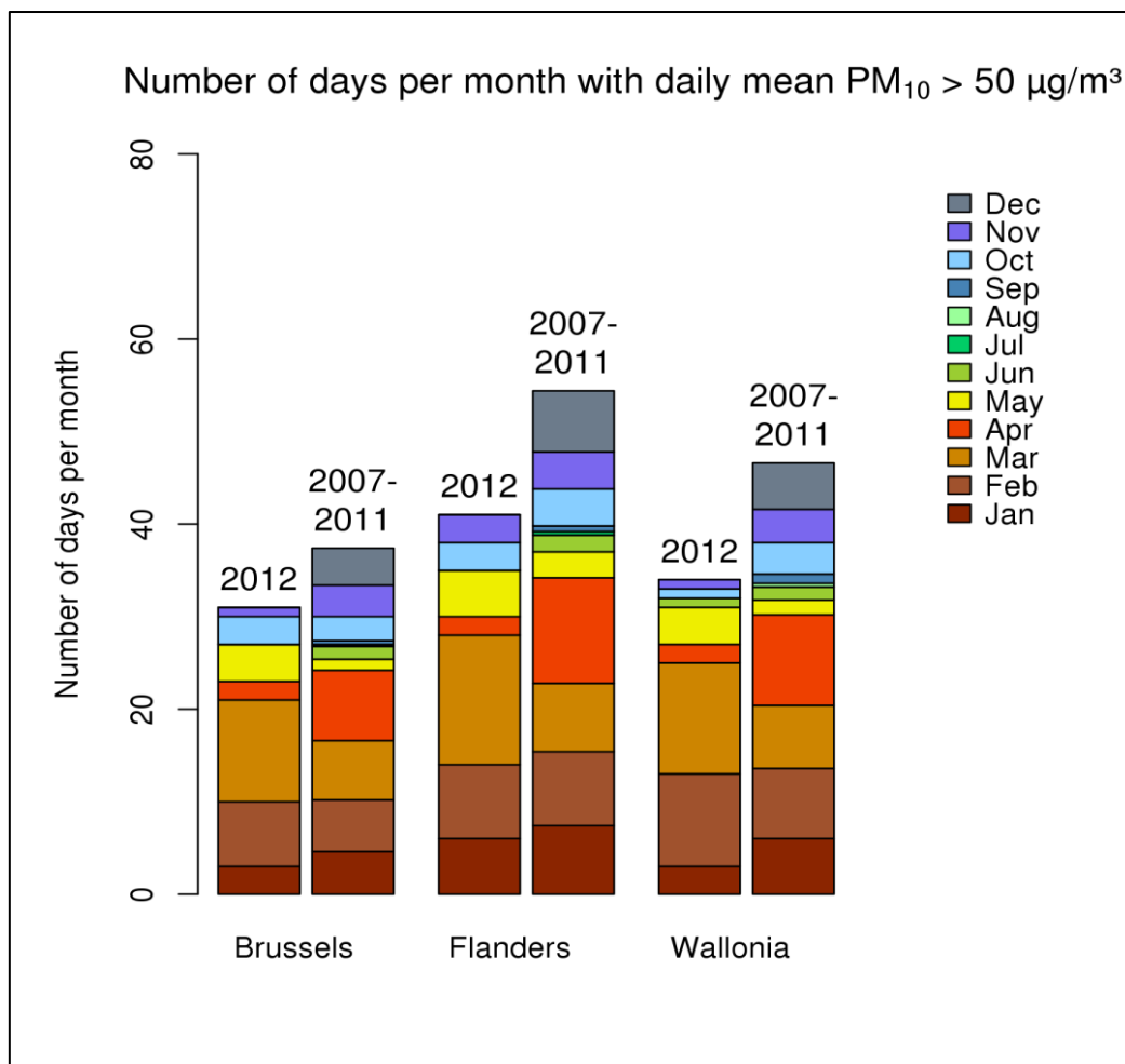
Figuur 18: Hoogste aantal dagen per maand waarop ergens in het Brussels Hoofdstedelijk, het Vlaams en het Waals Gewest de daggemiddelde grenswaarde van 50 \mu g/m^3 overschreden werd in 2012 en de drie voorgaande jaren. Alle data werden berekend op basis van de RIO-interpolatietechniek.
