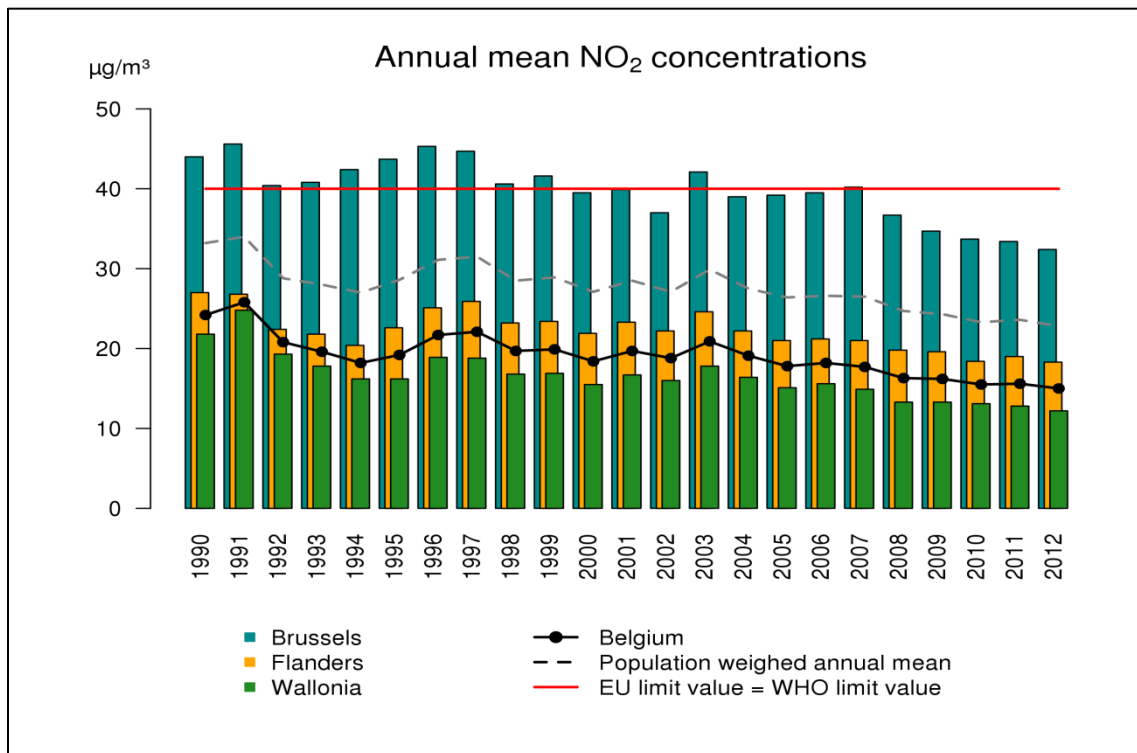
Figuur 29: Evolutie van het NO 2 -jaargemiddelde in België op basis van de RIO-interpolatietechniek.
