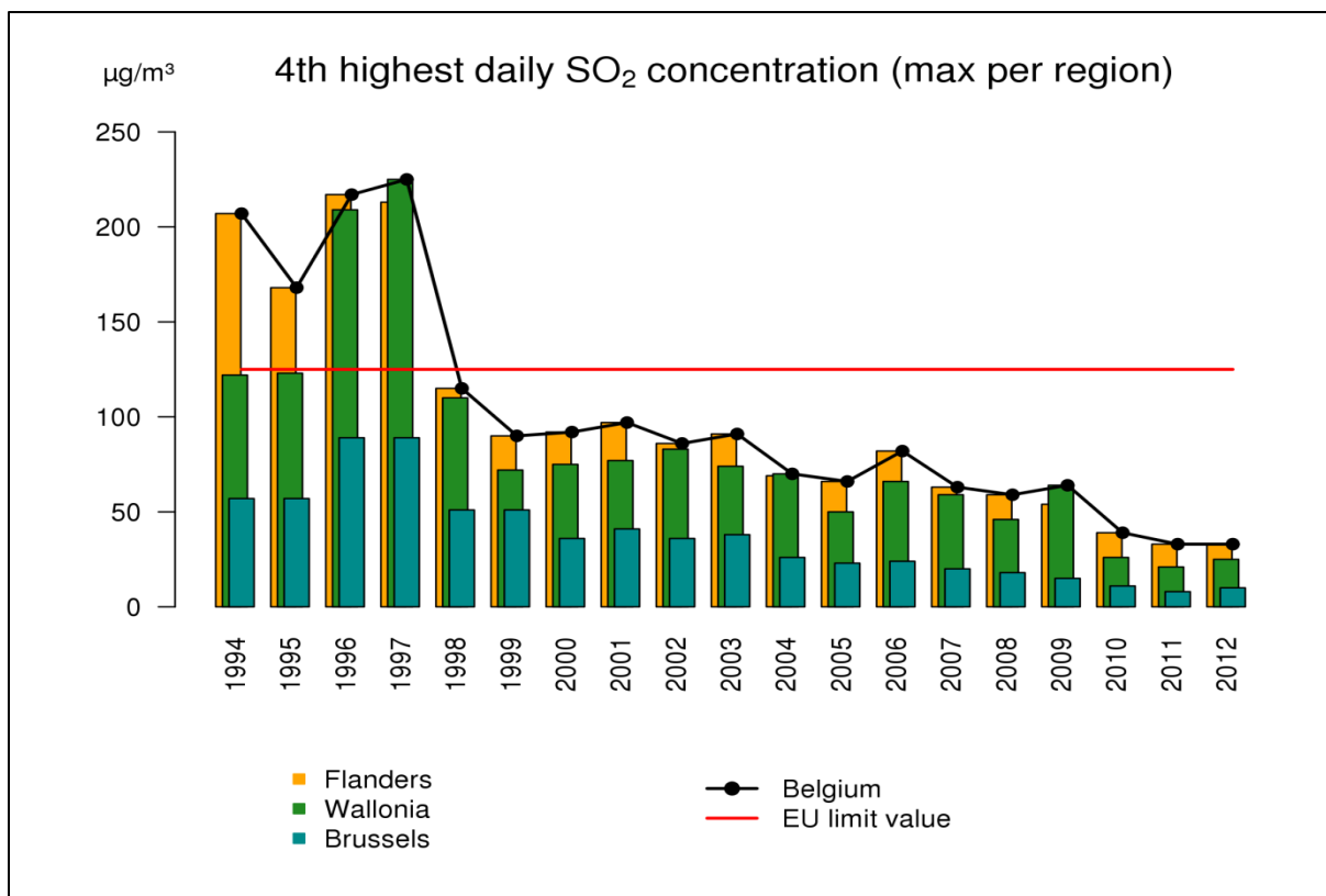
Figuur 56: Evolutie van de maximale 4e hoogste daggemiddelde SO 2 -concentratie per gewest en in België op basis van de RIO-interpolatietechniek.
