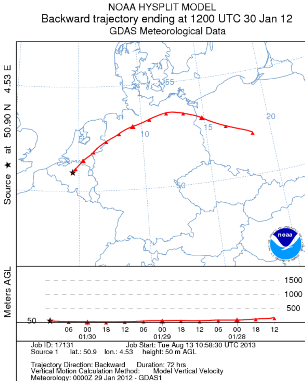
Figuur 4: Trajectbepaling van de luchtmassa die België bereikt op 30 januari 2012.
