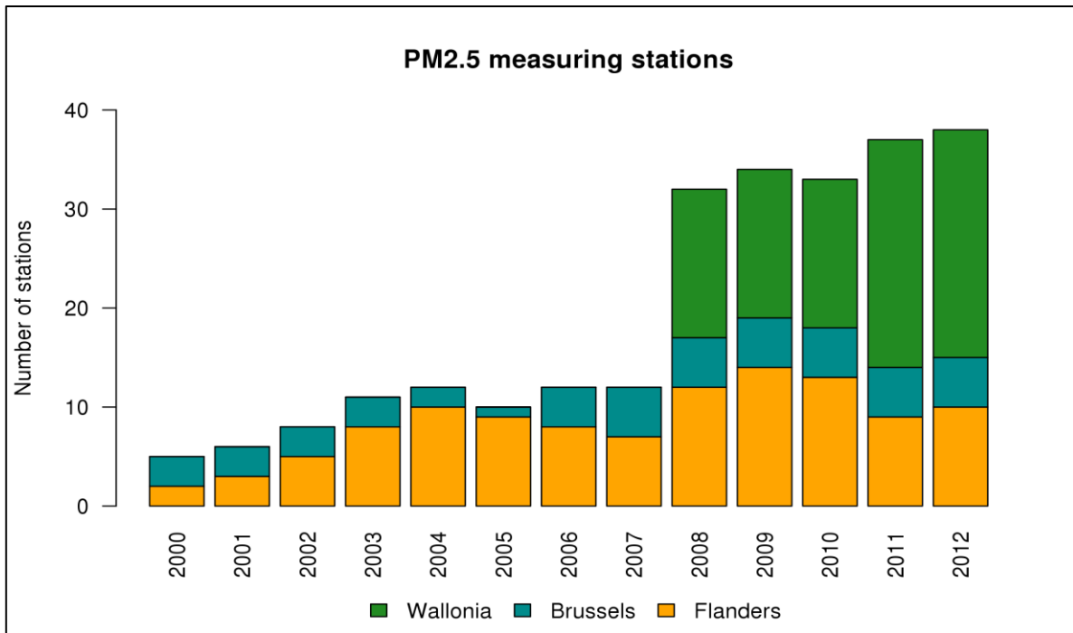
Figuur 19: Evolutie van het aantal PM 2,5 -meetstations in België.
