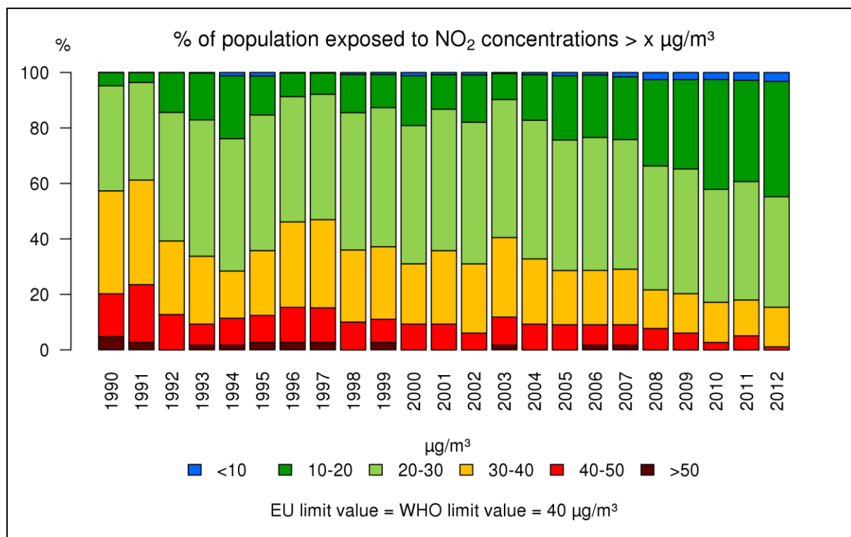
Figuur 31: Percentage van de Belgische bevolking blootgesteld aan jaargemiddelde \text{NO}_2 -concentraties. Alle data werden berekend op basis van de RIO-interpolatietechniek.
