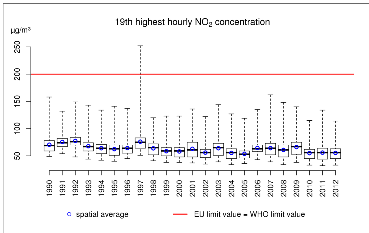
Figuur 33: Boxplot van de 19 de hoogste uurgemiddelde NO 2 -concentratie (µg/m 3 ) over de periode 1990-2012. Het ruimtelijke gemiddelde wordt door de blauwe cirkels weergegeven. Alle data werden berekend op basis van de RIO-interpolatietechniek.
