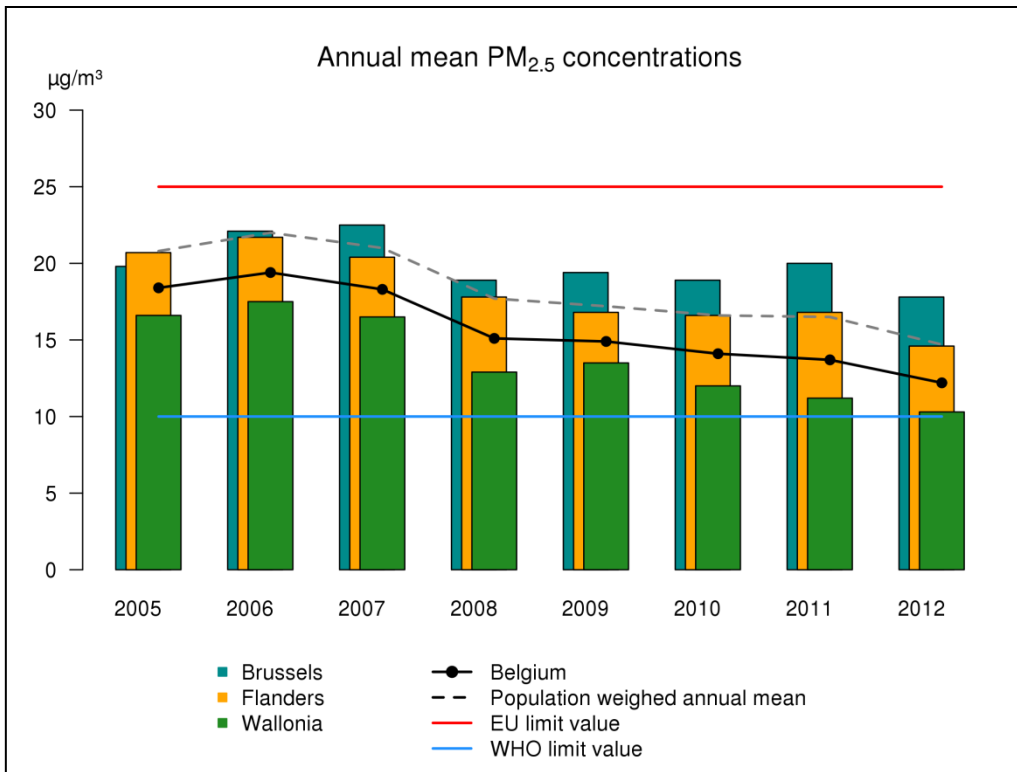
Figuur 22: Evolutie van de ruimtelijk jaargemiddelde PM 2.5 -concentraties voor de drie gewesten en België, en ook de bevolkingsgewogen jaargemiddelde concentratie voor België. Alle data werden berekend op basis van de RIO-interpolatietechniek.
