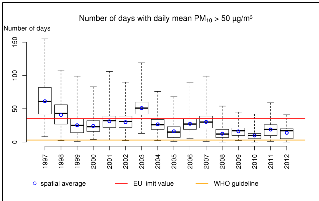
Figuur 14: Boxplot van het aantal dagen per jaar waarop de daggemiddelde PM_{10} -concentraties hoger was dan 50 \mu g/m^3 . Het ruimtelijk gemiddelde wordt weergegeven door de blauwe cirkels. Alle data werden berekend op basis van de RIO-interpolatietechniek.
