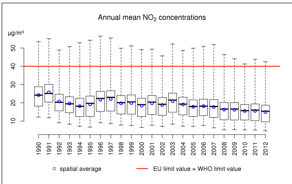
Figuur 28: Boxplots van de jaargemiddelde NO 2 -concentraties (µg/m 3 ) voor de periode 1990-2012. Het ruimtelijke gemiddelde wordt door de blauwe cirkels weergegeven. Alle data werden berekend op basis van de RIO-interpolatietechniek.
