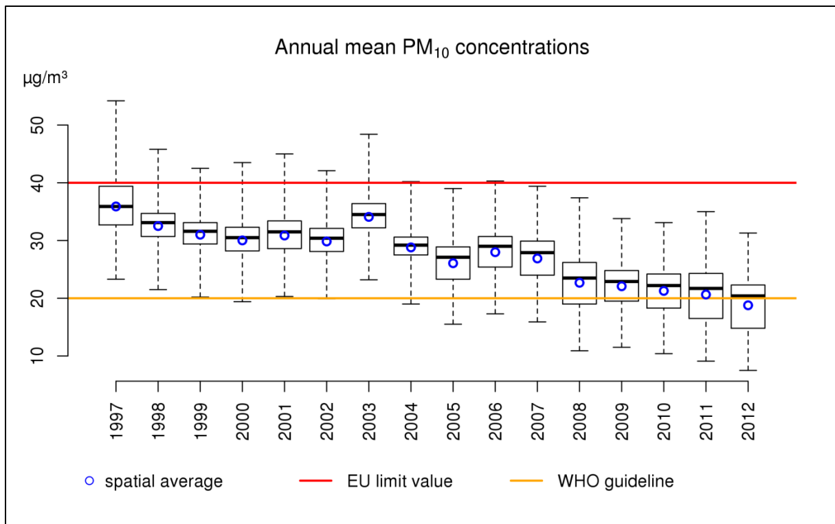
Figuur 9: Boxplot van de jaargemiddelde PM 10 -concentraties (µg/m 3 ) over de periode 1997-2012 in België. Het ruimtelijke gemiddelde wordt door de blauwe cirkels weergegeven. Alle data werden berekend op basis van de RIO-interpolatietechniek.
