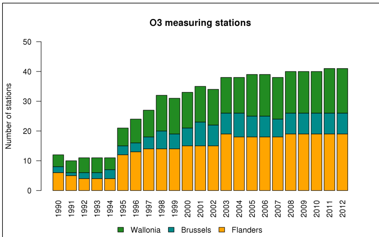
Figuur 35: Evolutie van het aantal O 3 -meetstations in België.
