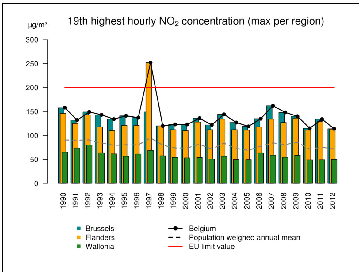
Figuur 34: Evolutie van het maximum van de 19 de hoogste NO 2 -uurwaarde in de drie gewesten en België op basis van de RIO-interpolatietechniek.
