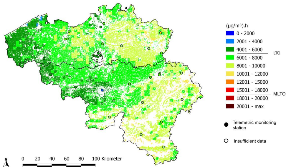
Figuur 42: Ruimtelijke spreiding van de overlast voor de vegetatie (AOT40 voor vegetatie), 2012. 'Insufficient data' betekent dat de data niet voldoen aan de criteria uit richtlijn 2008/50/EG annex VII voor het aggregeren van de meetgegevens. Alle data werden berekend op basis van de RIO-interpolatietechniek.
