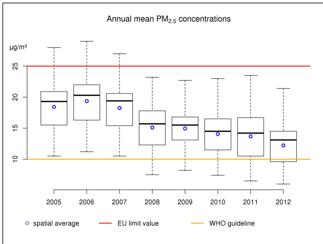
Figuur 21 Boxplot van de jaargemiddelde PM 2.5 -concentraties ( \mu\text{g}/\text{m}^3 ) over de periode 2005-2012. Het ruimtelijke gemiddelde wordt door de blauwe cirkels weergegeven. Alle data werden berekend op basis van de RIO-interpolatietechniek.
