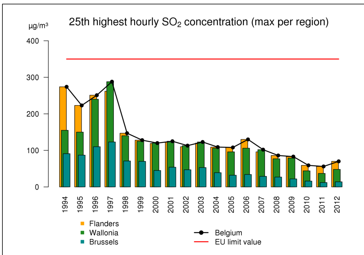
Figuur 54: Evolutie van de maximale 25e hoogste uurgemiddelde SO 2 -concentratie per gewest en België op basis van de RIO-interpolatietechniek.
