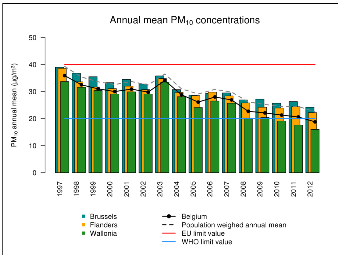
Figuur 10: Evolutie van de ruimtelijk gespreide jaargemiddelde PM 10 -concentratie in België en de drie gewesten, en het bevolkingsgewogen gemiddelde voor België. Alle data werden berekend op basis van de RIO-interpolatietechniek.
