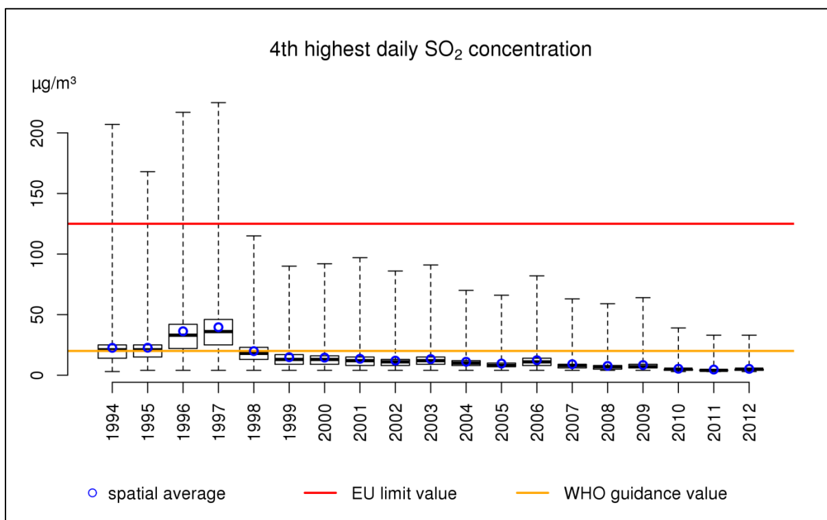
Figuur 57: Boxplot van de 4e hoogste daggemiddelde SO 2 -concentratie over de periode 1994-2012 over België op basis van de RIO-interpolatietechniek.
