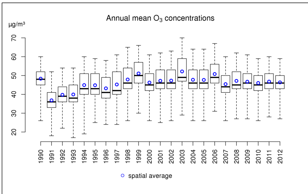
Figuur 49: Boxplot van jaargemiddelde O 3 -concentraties over de periode 1990-2012. Het ruimtelijk gemiddelde wordt weergegeven door de blauwe cirkels. Alle data werden berekend op basis van de RIO-interpolatietechniek.
