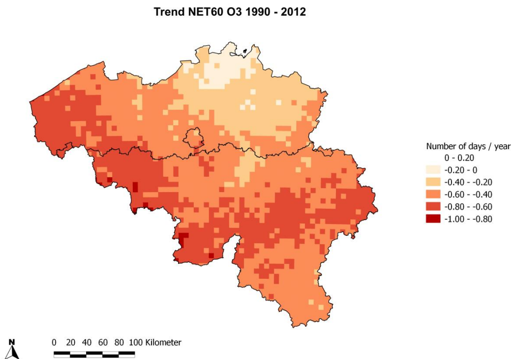
Figuur 39: Trend (aantal dagen/jaar) van het aantal dagen met de hoogste 8-uurgemiddelde ozonconcentratie boven 120 µg/m 3 (NET60) in de periode 1990-2012. Alle data werden berekend op basis van de RIO-interpolatietechniek.
