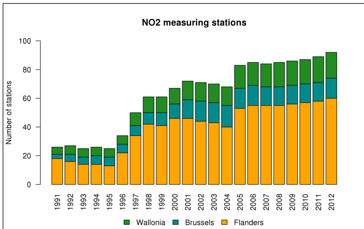
Figuur 25: Evolutie van het aantal NO 2 -meetstations in België.
