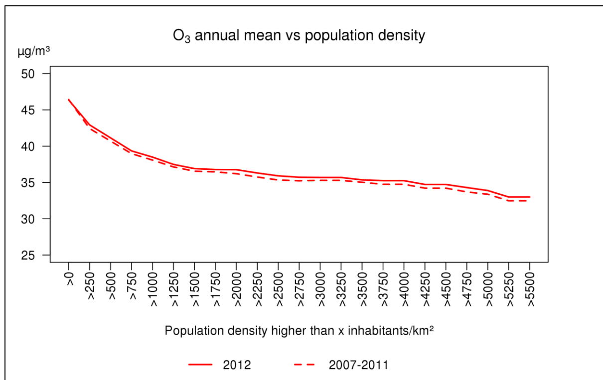
Figuur 48: Relatie tussen de geïnterpoleerde jaargemiddelde \text{O}_3 -concentraties op basis van de RIO-interpolatietechniek en de bevolkingsdichtheid (inwoners/ \text{km}^2 ).
