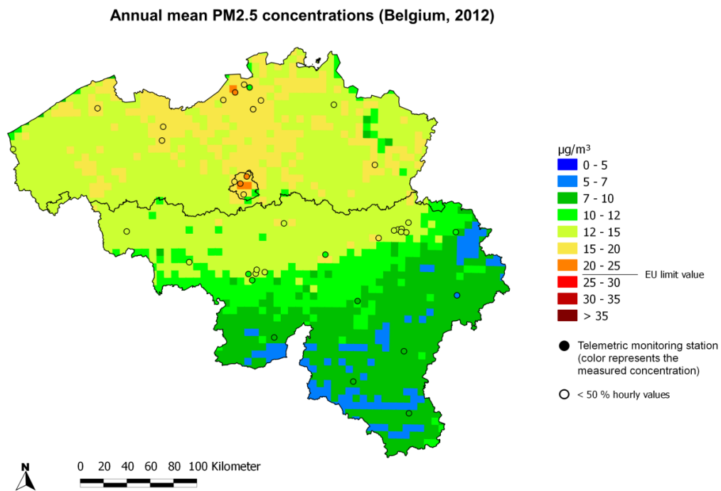
Figuur 20: Ruimtelijke spreiding van de jaargemiddelde PM 2.5 -concentratie in België in 2012. Alle data werden berekend op basis van de RIO-interpolatietechniek.
