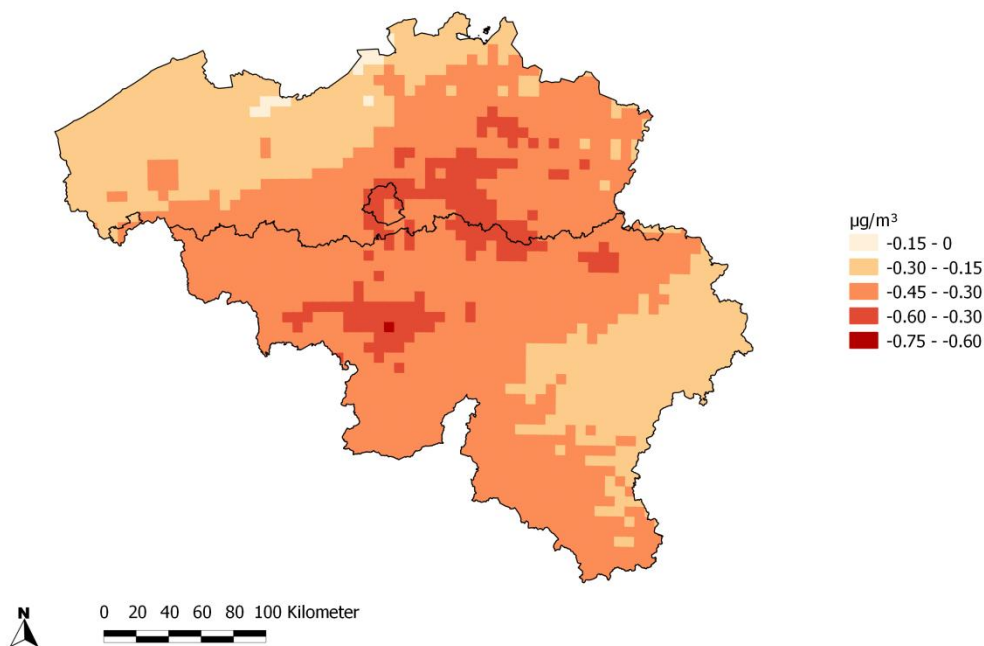
Figuur 30: Trend ( \mu\text{g}/\text{m}^3/\text{jaar} ) van de jaargemiddelde \text{NO}_2 -concentraties in de periode 1990-2012. Alle data werden berekend op basis van de RIO-interpolatietechniek.
