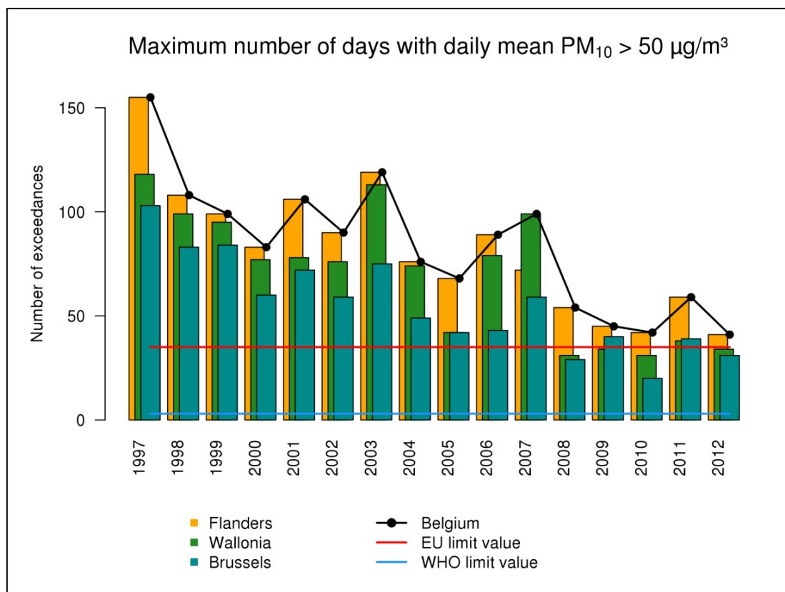
Figuur 15: Evolutie van het maximale aantal dagen per jaar waarop de daggemiddelde PM_{10} -concentratie hoger was dan 50 \mu g/m^3 in België en de drie gewesten. Alle data werden berekend op basis van de RIO-interpolatietechniek.
